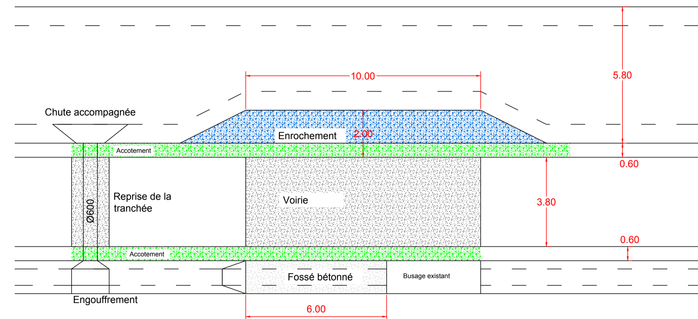
Vue en plan Reprise de la voirie et renforcement de berge du canal
